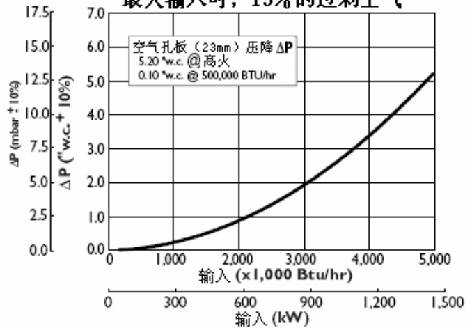
空气孔板压降 与输入之间的关系 (在测压口A与C之间测量) 最大输入时，15%的过剩空气
