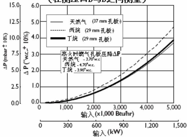
燃气孔板压降 \Delta P 与输入之间的关系 (在测压口B与D之间测量)
